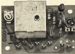
Görler-Rauschperre (14) »Typ 326-0010«
