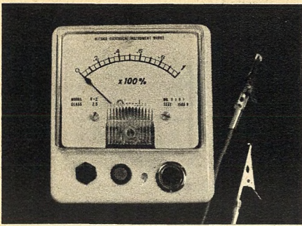
Bild 3. Ansicht des fertigen Gerätes
