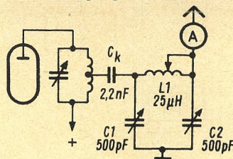
Bild 9. Schaltung eines Collins-Filters (Pi-Filters) zum Anpassen von Linear-Allbandantennen an Sender-Endstufen
