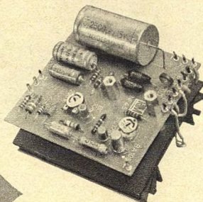
(8) »BG 40«
