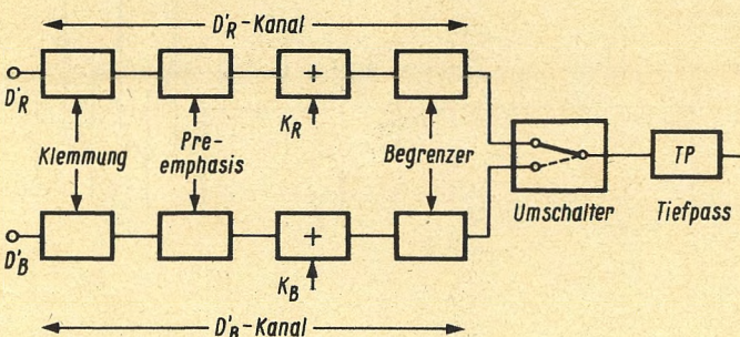
Bild 2. Blockschaltbild für die niederfrequente Aufbereitung der FD-Signale
