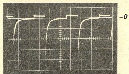
Bild 8. Spannung am Gate des Thyristors GTO. Maßstab: vertikal 5 V/T, horizontal 20 μs/T
