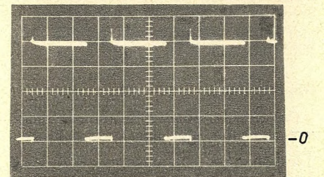
Bild 10. Spannung an der Anode des Thyristors GTO. Maßstab: vert. 100 V/T, horiz. 20 μs/T
