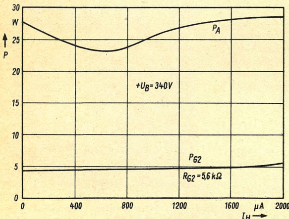
Bild 24. Anoden- und Schirmgitterverlustleistung einer Röhre PL 509 in einer mit diesem Netzteil betriebenen Horizontal-Endstufe für 110^\circ -Farbbildröhre in Abhängigkeit vom Strahlstrom
