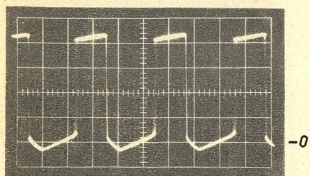
Bild 6. Spannung am Kollektor des Transistors T 1. Maßstab: vertikal 2 V/T, horizontal 20 μs/T
