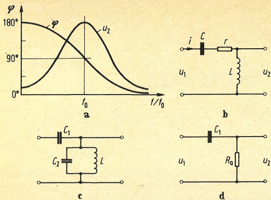
▲ Bild 3. a = Amplituden- und Phasengang von Schwingkreisen in Vierpolschaltung. Bei der Resonanzfrequenz f_0 beträgt der Phasenwinkel der Ausgangsspannung 90^\circ ; b = Serienschwingkreis als Vierpol; c = Parallelschwingkreis mit kleinem Vorschaltkondensator C_1 als Vierpol; d = Ersatzschaltung zu Bild 3c
