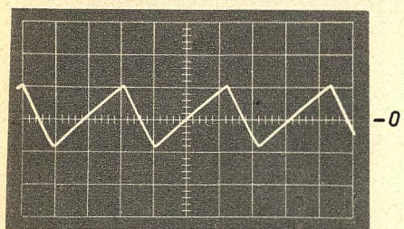
Bild 5. Spannung am Emitter des Transistors T 1. Maßstab: vertikal 1 V/T, horizontal 20 μs/T
