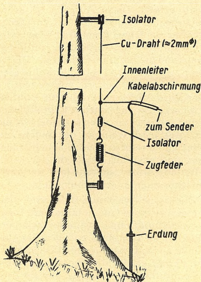
Bild 7. Vertikal-Longdrahtantenne, an einem Baum verspannt
