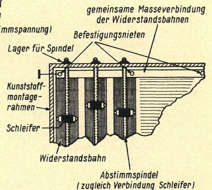
▶ Bild 2. Mechanische und elektrische Ausführung der elektronischen Abstimmung
