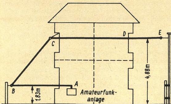
▲ Bild 1. Langdrahtantenne für Dachbodenmontage mit Ableitung zur Hausmitte
