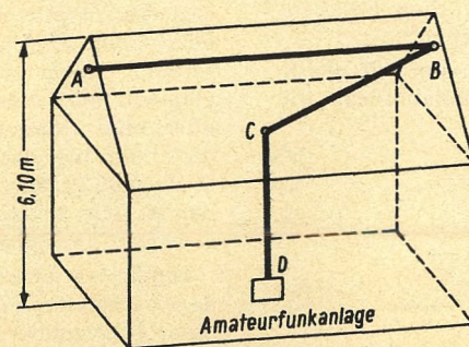
▲ Bild 1. Langdrahtantenne für Dachbodenmontage mit Ableitung zur Hausmitte
