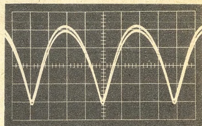
Bild 20. Parabelförmig modulierte Ausgangsspannung des Netzteiltes. Maßstab: vertikal 10 V/T, horizontal 5 ms/T
