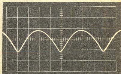
Bild 19. Integrierte Vertikalspannung als Führungsgröße für den Regelkreis (Punkt F). Maßstab: vertikal 2 V/T, horizontal 5 ms/T
