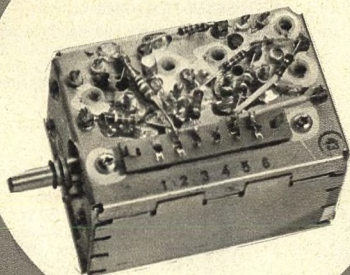
Görler-FET-Tuner (10) »Typ 312-2433«
