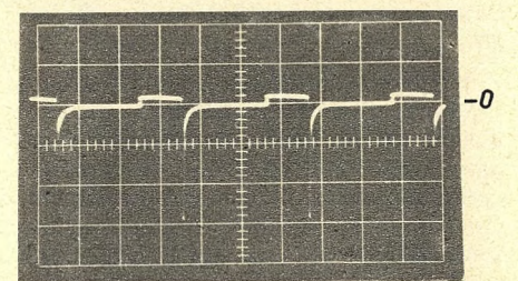
Bild 9. Gate-Strom des Thyristors GTO. Maßstab: vert. 1 A/T, horiz. 20 μs/T (neg. Spitzenwert = 3 A)
