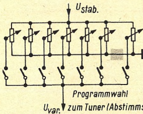
▶ Bild 2. Mechanische und elektrische Ausführung der elektronischen Abstimmung
