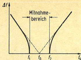
◀ Bild 7. Synchronisierungsbereich eines mitgezogenen Oszillators
