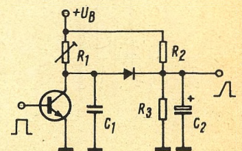
Bild 4. Schaltung zur Erzeugung von Kennimpulsen
