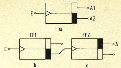
▲ Bild 11. Kurzzeichen für Flipflop-Stufen
