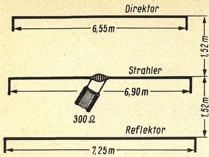
Bild 5. Drei-Element-Einband-Beam für Innenräume
