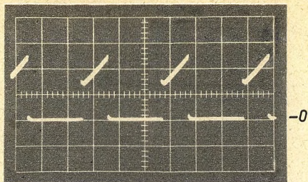
Bild 11. Anodenstrom des Thyristors GTO. Maßstab: vertikal 0,2 A/T, horizontal 20 \mu s/T
