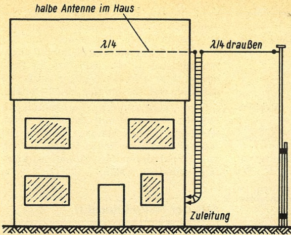
◀ Bild 6. Dipol- antenne, teilweise im Dachboden verspannt
