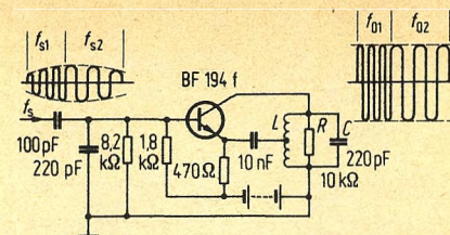
Bild 8. Prinzip eines mitgezogenen Oszillators. Die Oszillatorfrequenzen f_{01} und f_{02} werden durch die Steuerfrequenzen f_{s1} und f_{s2} synchronisiert
