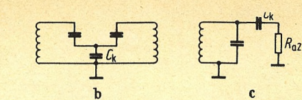
▲ Bild 5. a und b = kapazitiv gekoppelte Bandfilter; c = Ersatzschaltung
