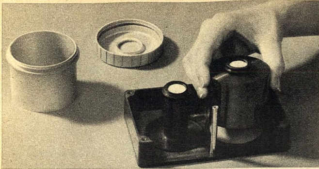
▲ Bild 1. Diese kleine Ampex-Kassette nimmt ein 2-Zoll-Magnetband für eine Spielzeit von 10 s auf, ausreichend für Werbespots oder sonstige kurze Einblendungen in das Fernsehprogramm. Bei Nichtgebrauch oder für den Postversand wird der Bandwinkel in dem leichten Behälter links untergebracht
