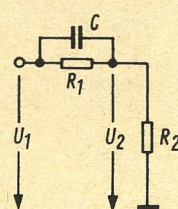
Bild 3. Schaltung für die Preemphasis
