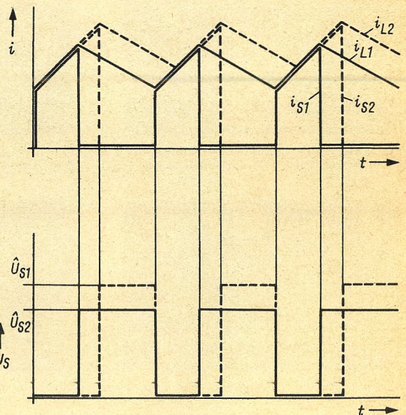
Bild 2. Strom, der über den Schalter S fließt
