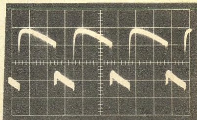
Bild 17. Zeilenfrequenter Anteil der Ausgangsspannung des Netzteiltes bei 80 W Belastung. Maßstab: vertikal 1 V/T, horizontal 20 \mu s/T
