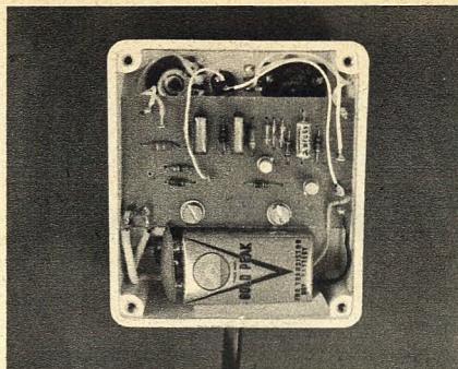
Bild 4. Innenaufbau des Schließwinkelmeßgerätes
