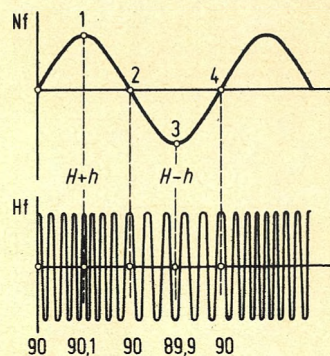
Bild 6. Umsetzen einer Tonfrequenzschwingung in Frequenzmodulation
