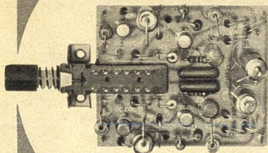
Stereo-Vorverstärker
