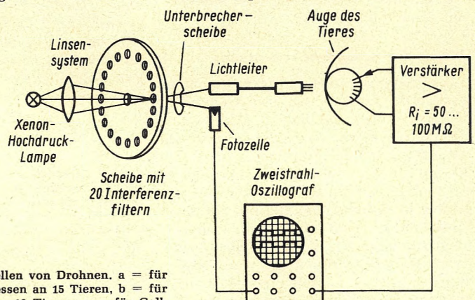
Bild 2. ► Meßeinrichtung zum Bestimmen der Farbempfindlichkeit von Sehzellen
