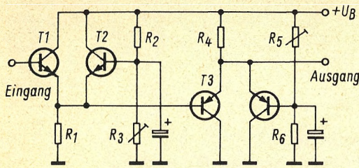
◀ Bild 5. Begrenzerschaltung mit einstellbarem unteren und oberem Begrenzungsniveau
