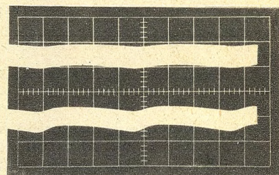
Bild 16. Netzfrequenter Restbrumm am Ausgang des Netzteiltes bei 80 W Belastung. Maßstab: vertikal 1 V/T, horizontal 5 ms/T
