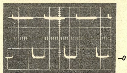
Bild 7. Basisspannung von Transistor T 3. Maßstab: vertikal 1 V/T, horizontal 20 μs/T
